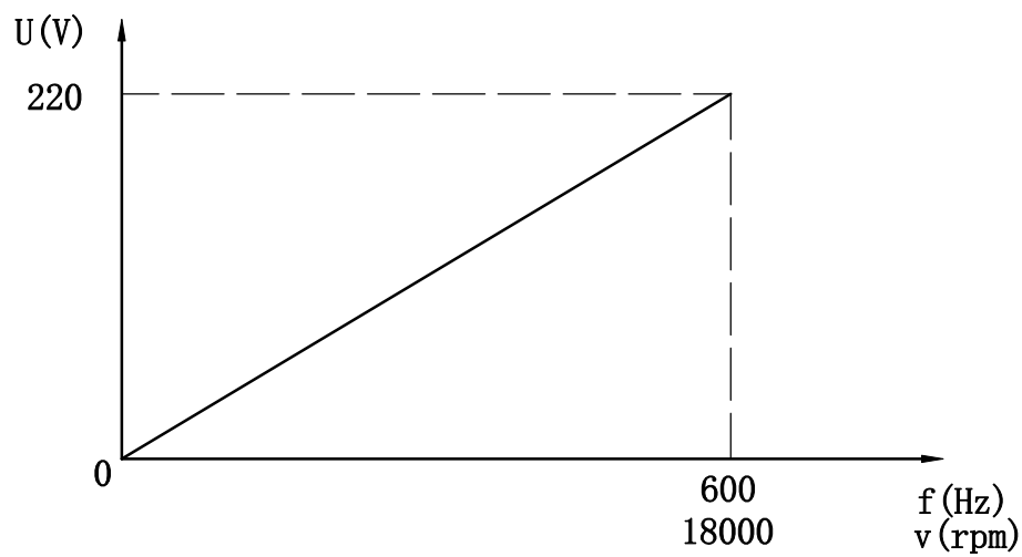
频压曲线 U. f Curve
