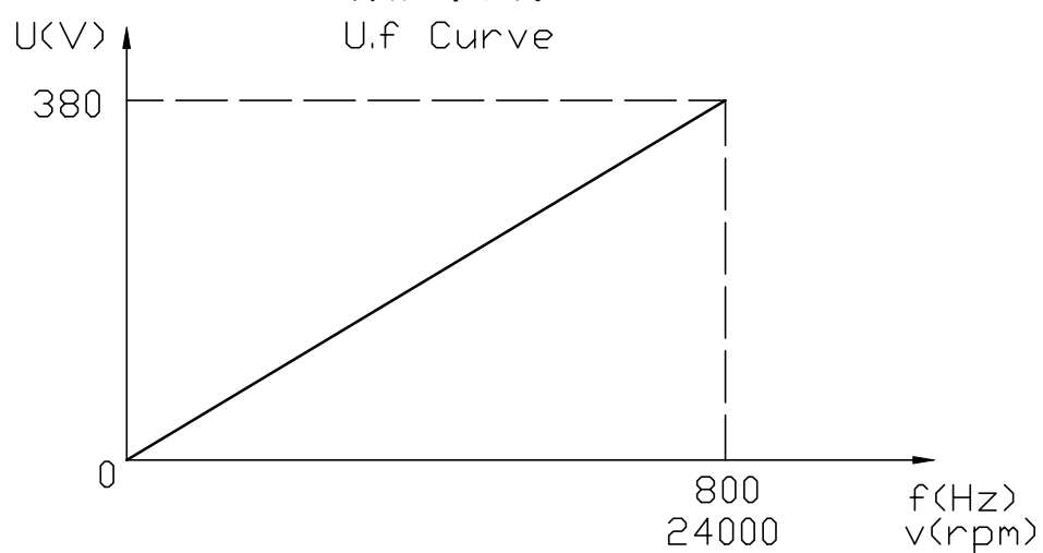
频压曲线
