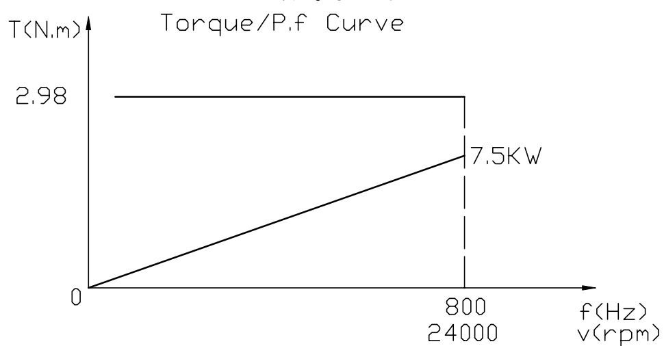
扭矩/功率曲线
