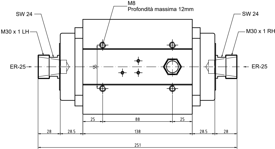
GDR51-18Z/2.2S Y380V/Δ220V 外形图
