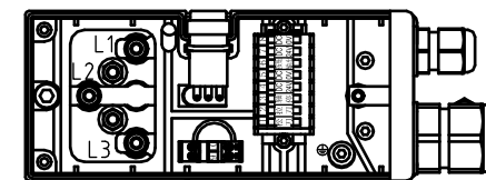
A向接线盒内
