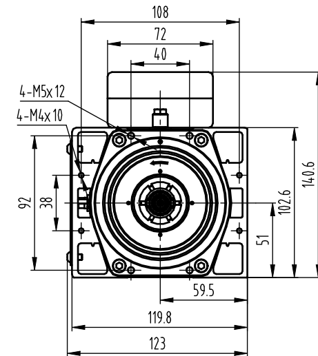
A向接线盒内
