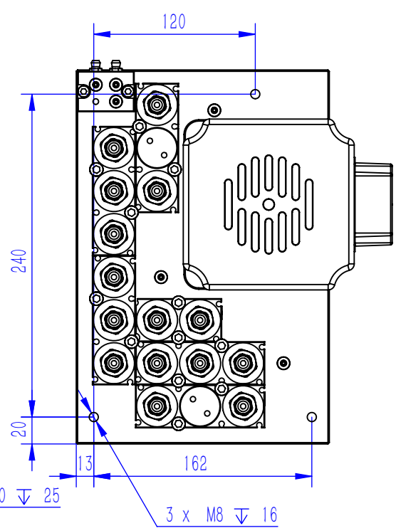
视图 B
