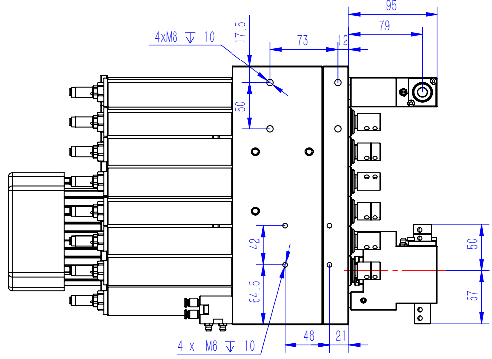
视图 B
