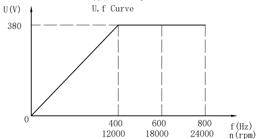
频压曲线
