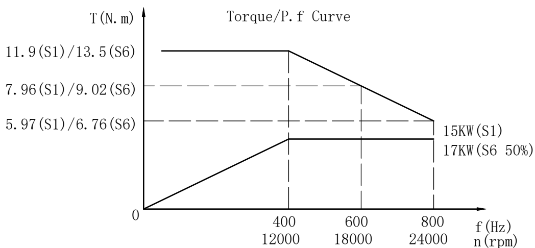
扭矩/功率曲线
