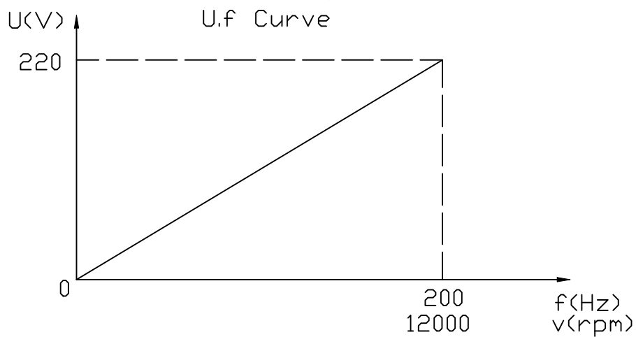
频压曲线
