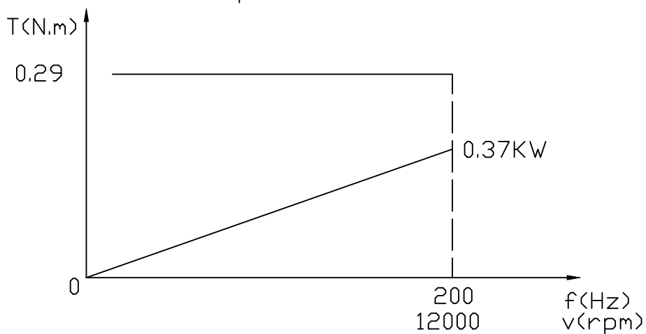
扭矩/功率曲线
